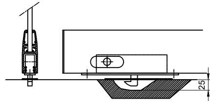
ABLOY LC306 + ME202 INTIGRERAD
